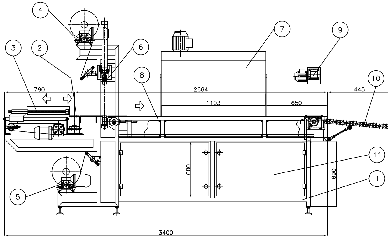
TERMOPAK 650
